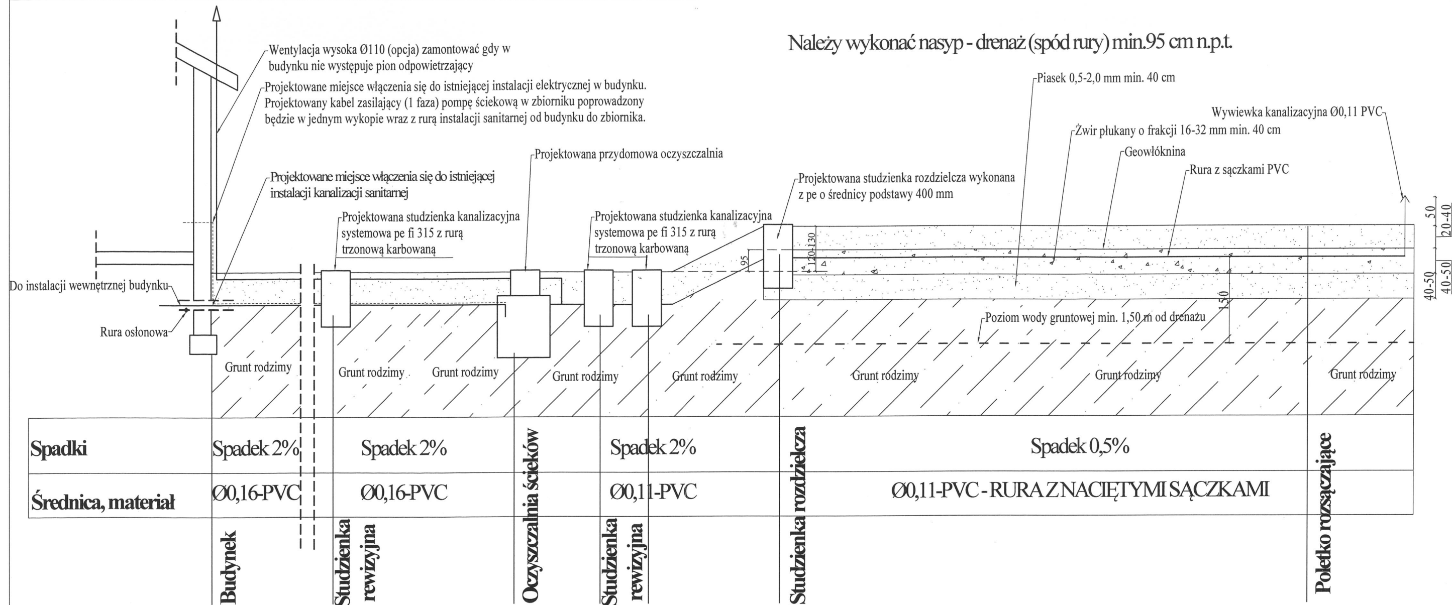
Drenaż rozsączający
