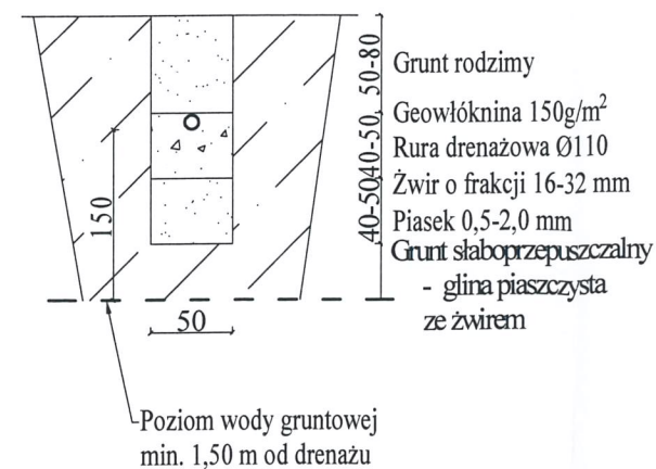
Przekrój wykopu pod drenaż
