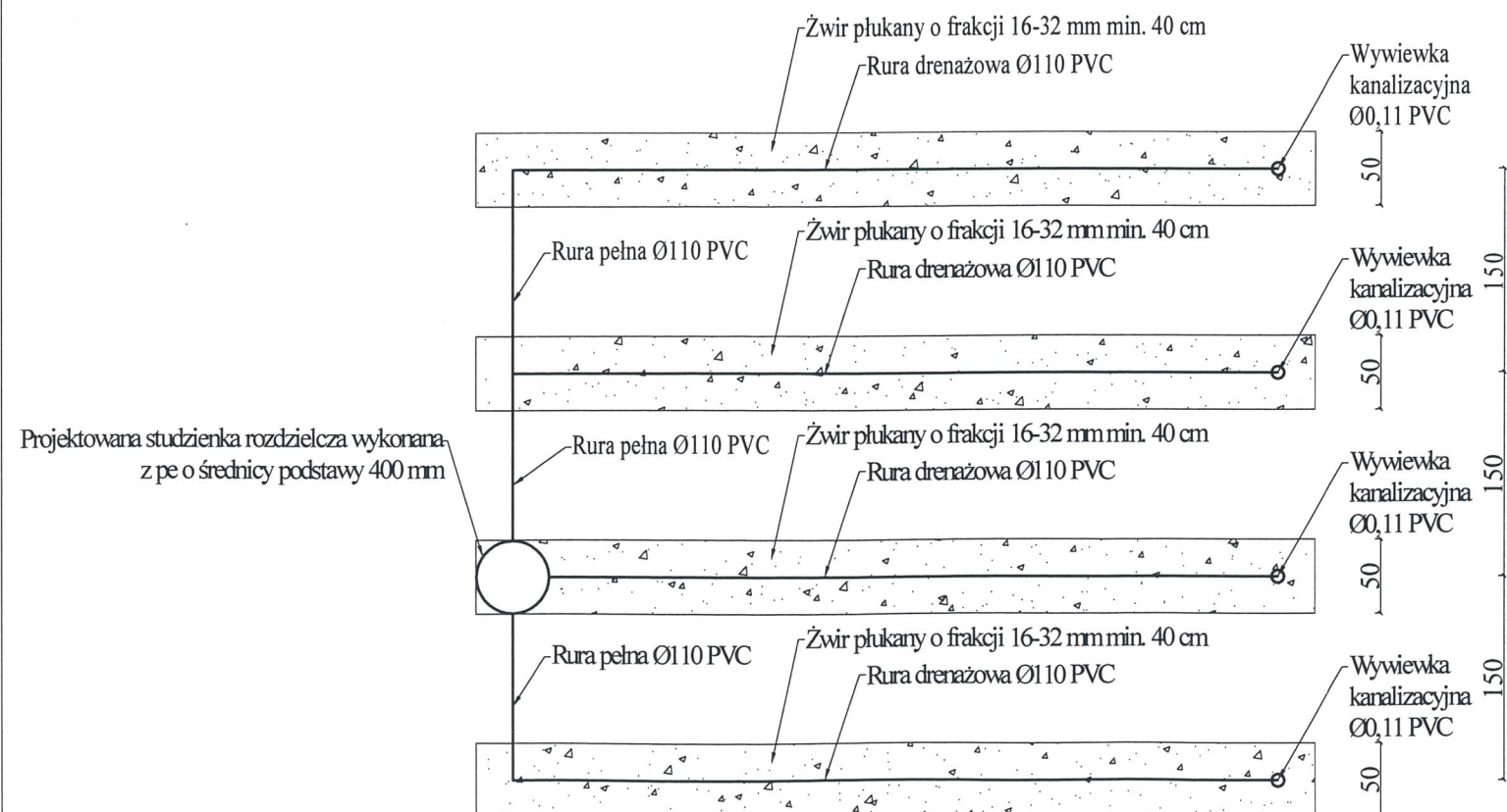
Drenaż rozsączający
