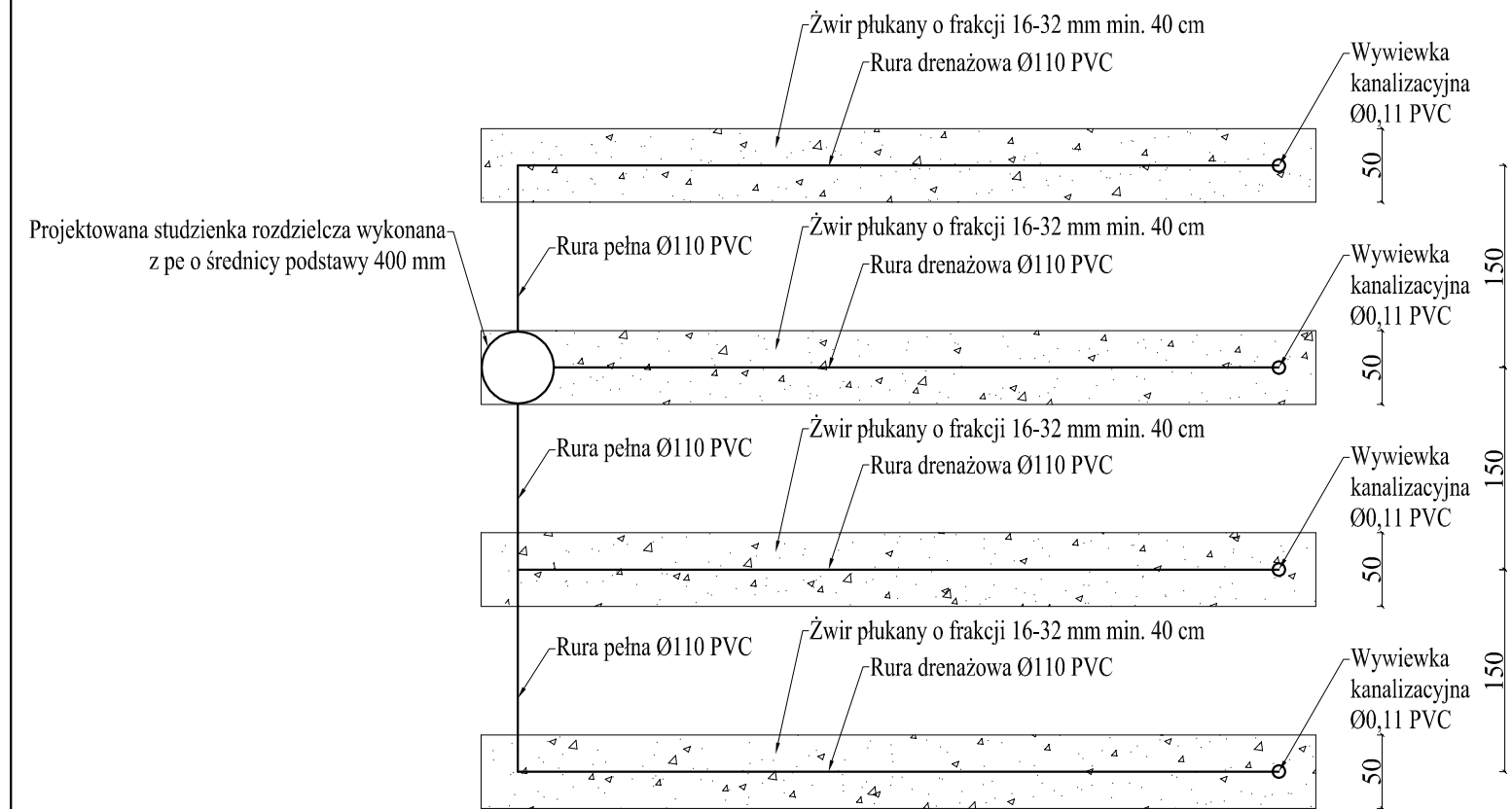
Drenaż rozsączający
