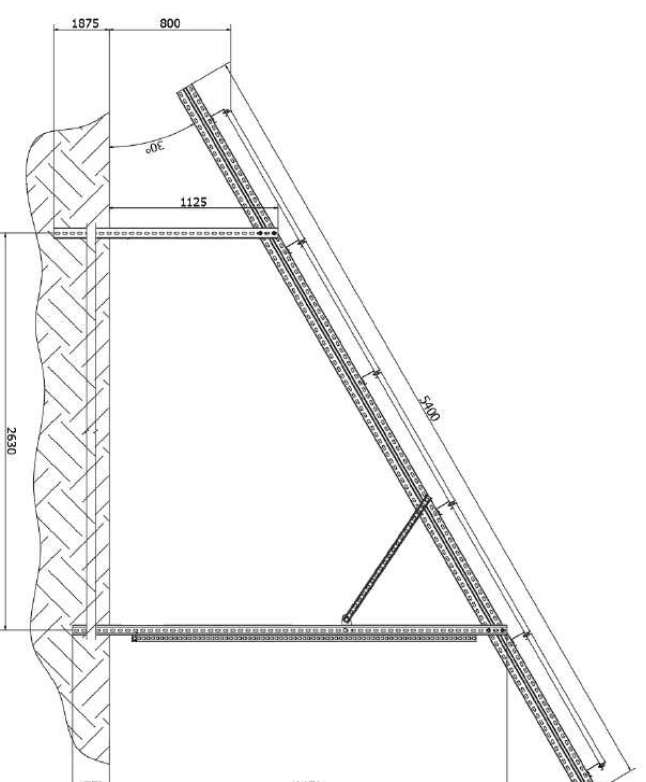
PRZEKRÓJ 1:50
